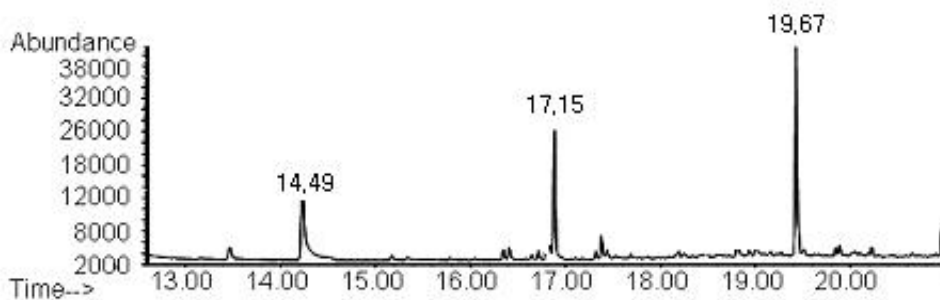
그림 13 지오스민, 2-MIB의 GC-MS 크로마토그램(예)
